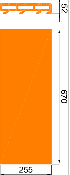
dettaglio lastra
