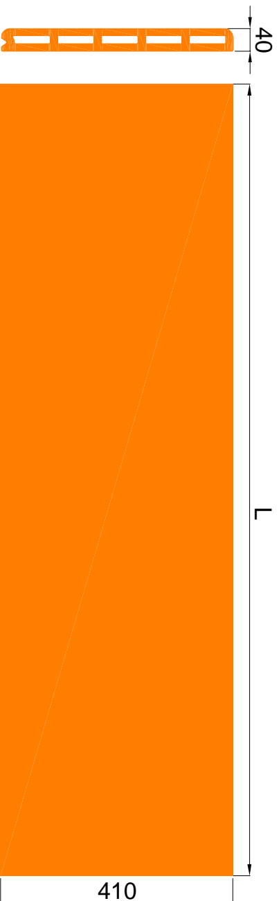
dettaglio lastra
