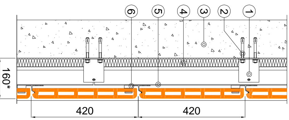
sezione verticale
