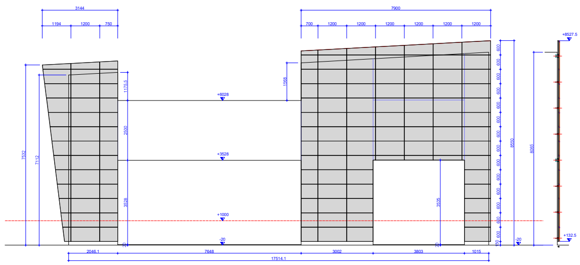
PROSPETTO NORD
