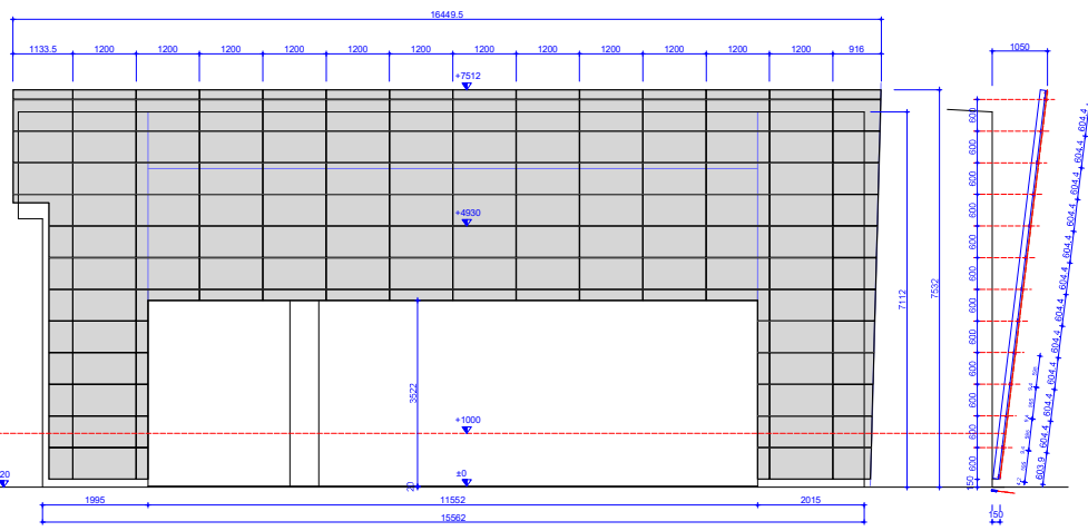
PROSPETTO EST
