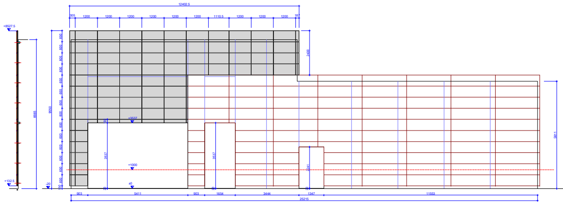
PROSPETTO OVEST
