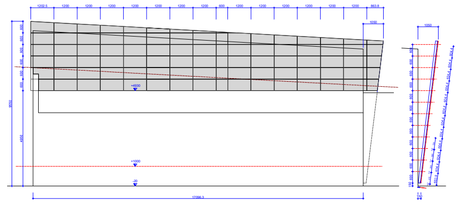
PROSPETTO SUD
