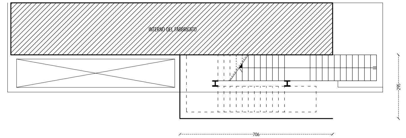
PLANIMETRIA - STATO DI PROGETTO
