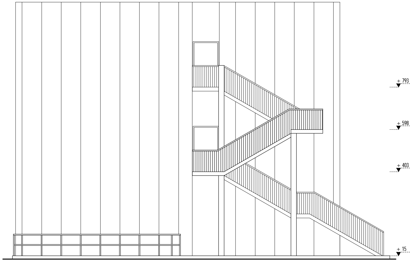
PROSPETTO - STATO DI FATTO
