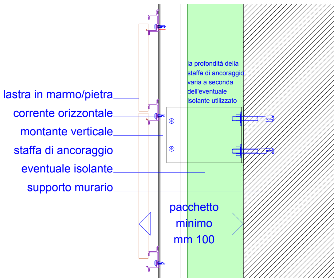
SEZIONE
