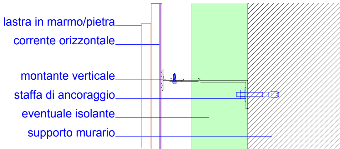
PIANTA
