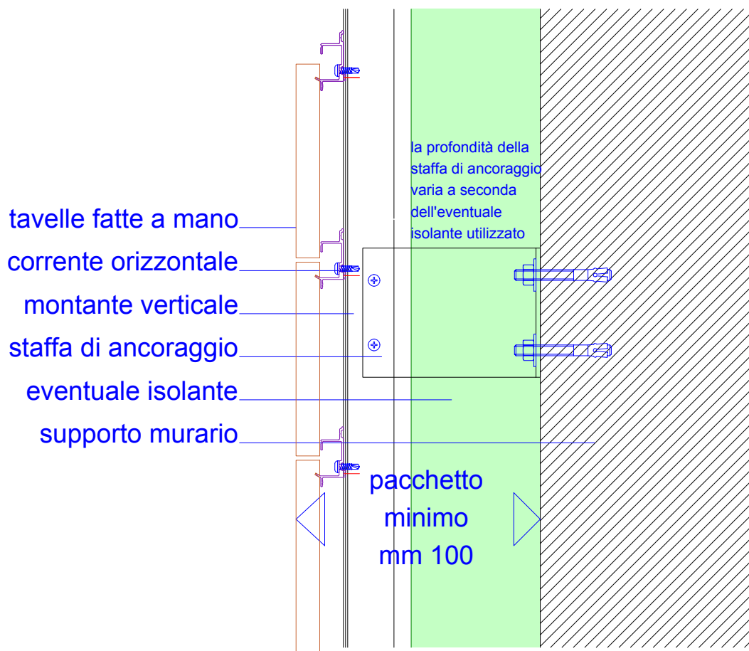
SEZIONE
