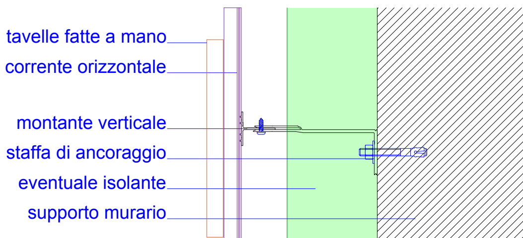
PIANTA
