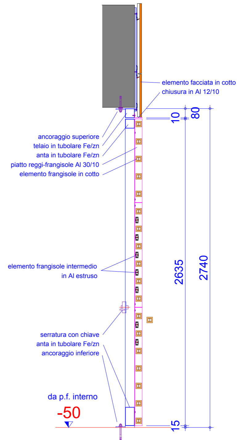
SEZIONE
