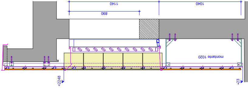
sezione finestra
