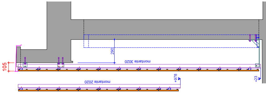
sezione rivestimento a tutta altezza
