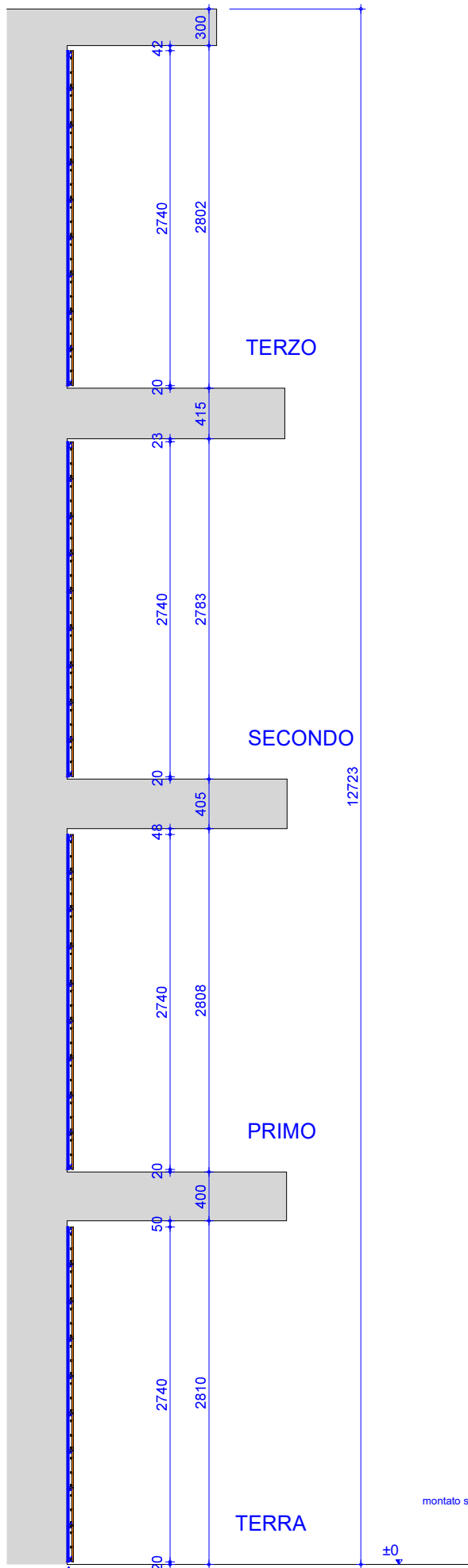
SEZIONE - LATO SUD
